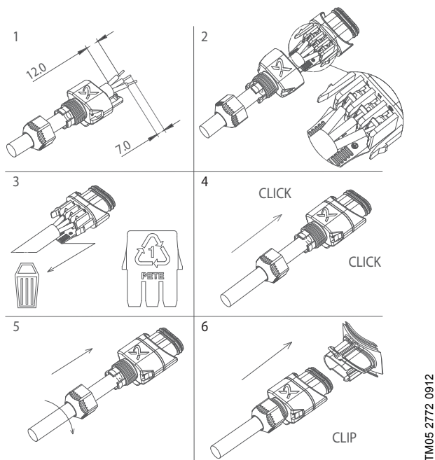
Рис. 10 Установка электроразъема
