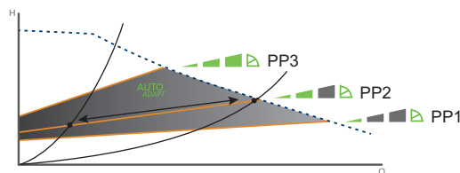
Рис. 15 Три кривые/настройки пропорционального регулирования
