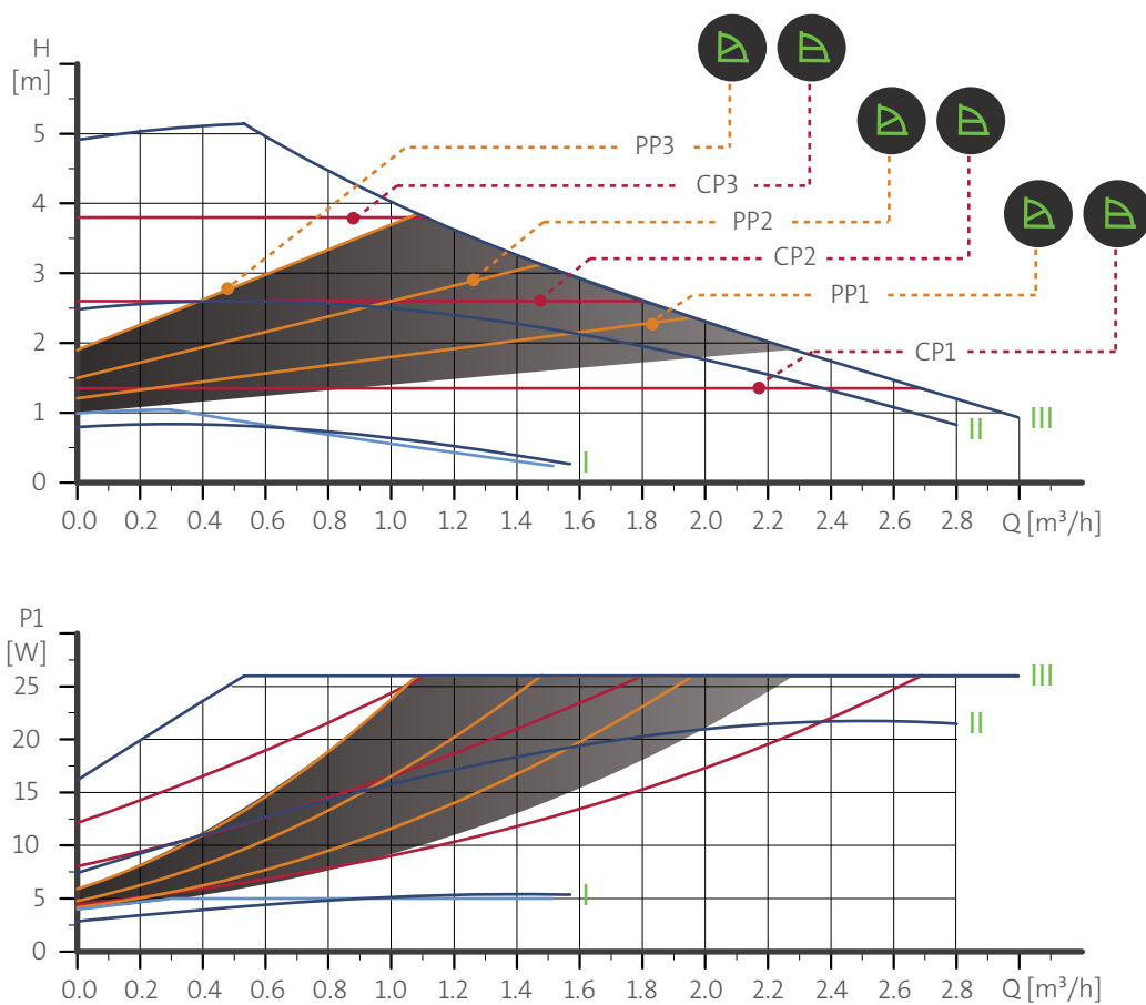
Рис. 31 ALPHA2 XX-50
